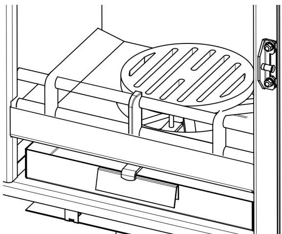
Bild 5 Rüttelrost
