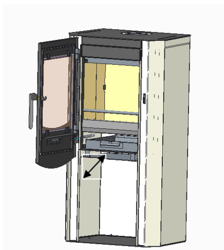
Bild 6 – Aschekasten
