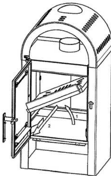
Bild 5 – Rost
