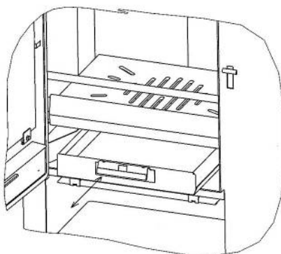
Bild 6 – Aschekasten
