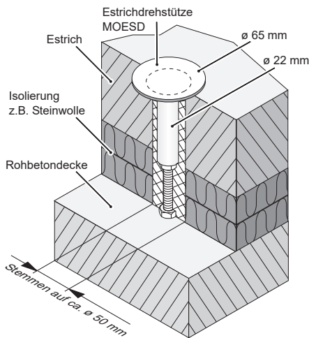
Aufbau bei schwimmenden Estrich mit Fußbodenheizung
