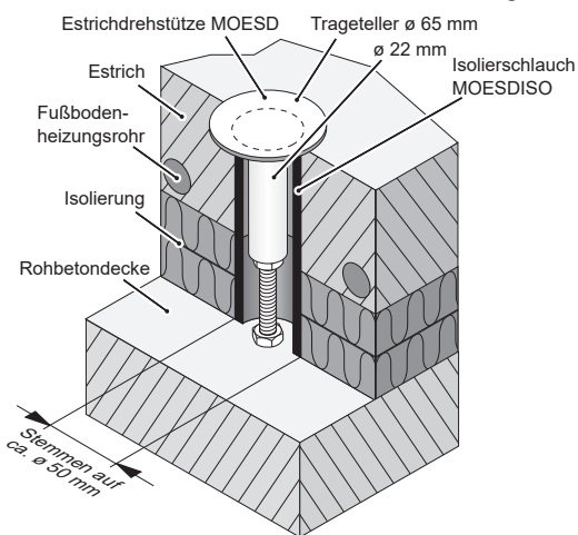
Aufbau bei schwimmenden Estrich mit Fußbodenheizung
