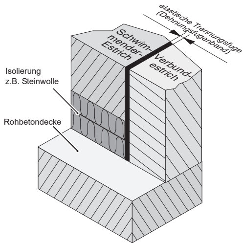
Aufbau bei schwimmenden Estrich und Verbundestrich
