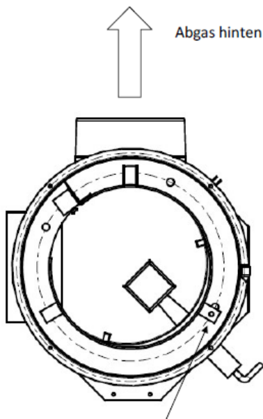
Bolzen
